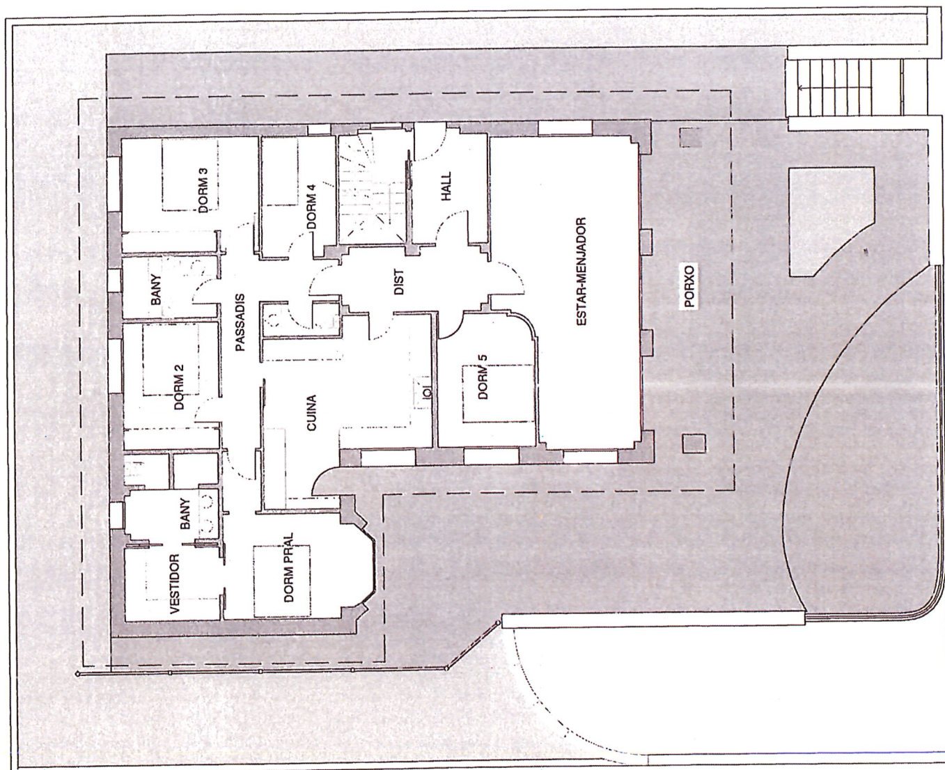
PLANTA BAIXA
